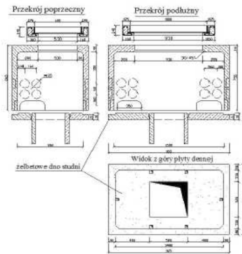
KONSTRUKCJA
